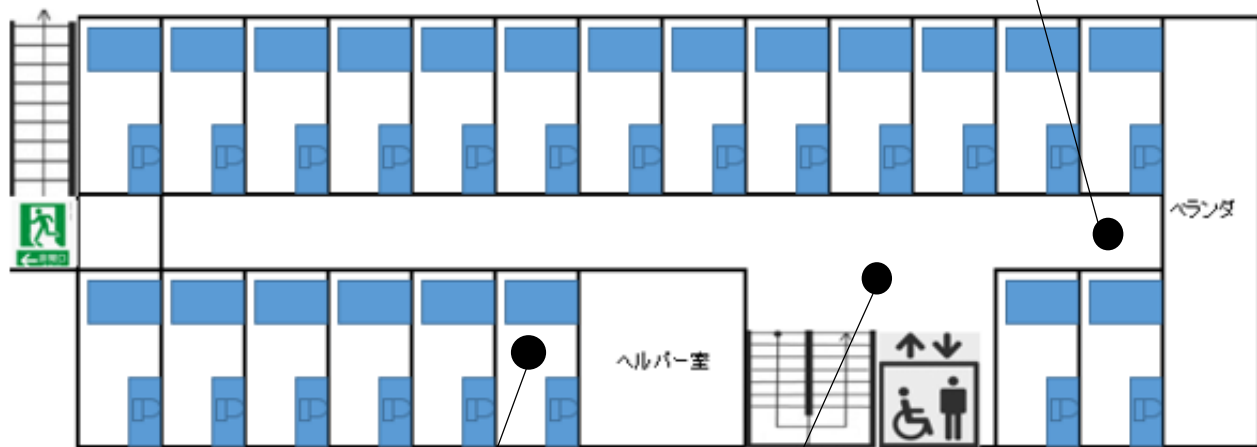
ライフパートナーこもれび 見取図 2F
